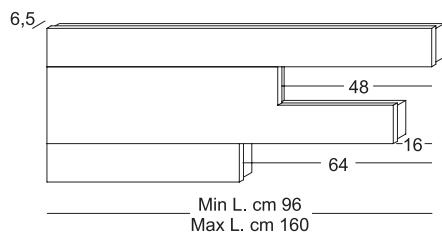
TESTATA ANGOLARE "B" L. cm 160 riducibile senza sovrapprezzo Min. cm 96
