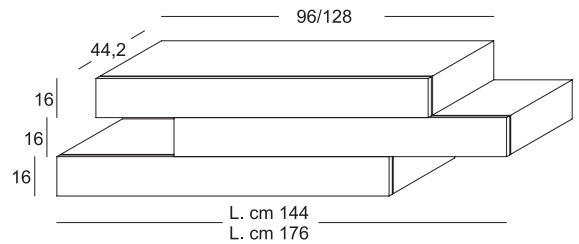
L. cm 144 cassetti L. cm 96
