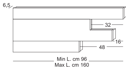
TESTATA ANGOLARE "A" L. cm 160 riducibile senza sovrapprezzo Min. cm 96
