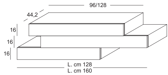
L. cm 128 cassetti L. cm 96
