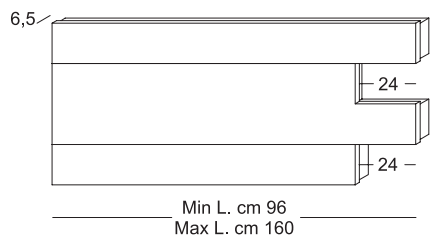
TESTATA ANGOLARE "C" L. cm 160 riducibile senza sovrapprezzo Min. cm 96
